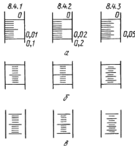
а — схема градуировки 1 (см. п. 8.3.1); б — схема градуировки 2 (см. п. 8.3.2); в — схема градуировки 3 (см. п. 8.3.3)
